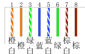
T568B的水晶头压法
